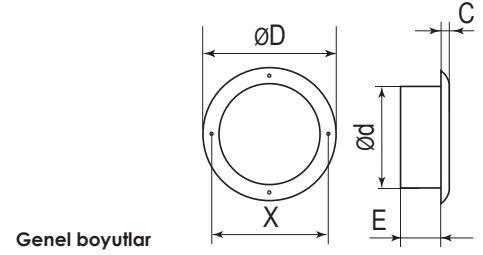
Genel boyutlar
