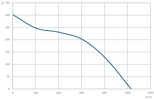
KAP 200
