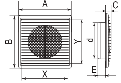
Genel boyutlar
