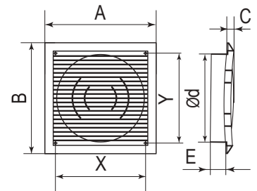
Genel boyutlar
