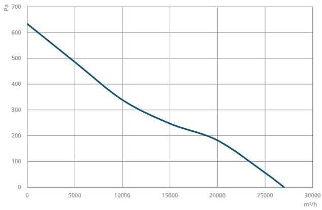
BAXI 800-5-35
