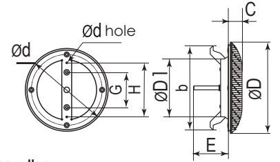
Genel boyutlar
