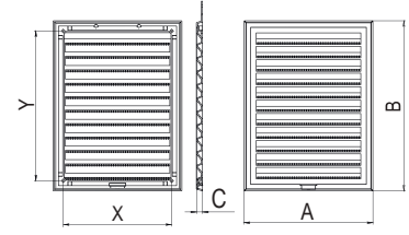
Genel boyutlar
