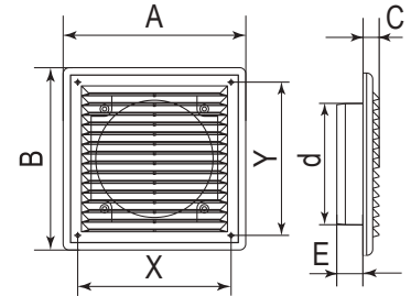
Genel boyutlar
