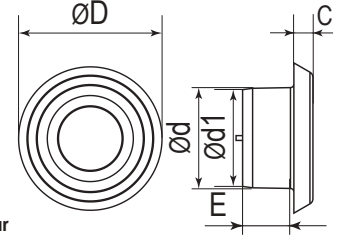
Genel boyutlar
