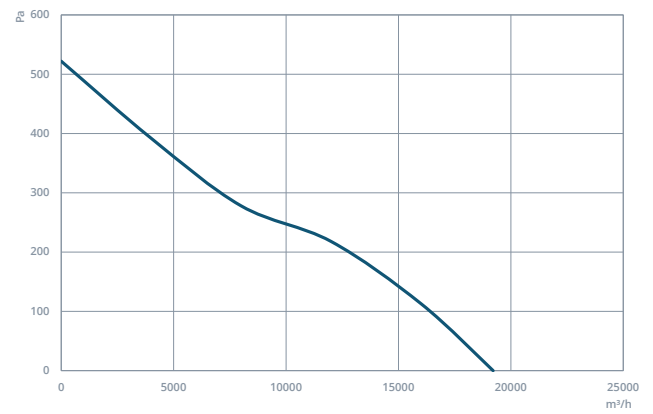
AXIP 710-5-30
