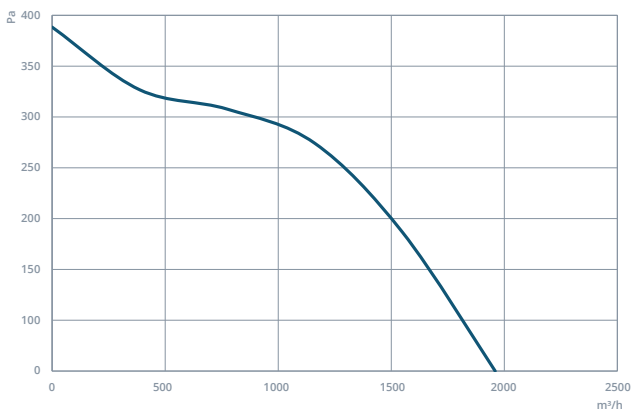
KAP 315
