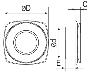
Genel boyutlar
