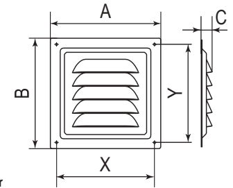
Genel boyutlar
