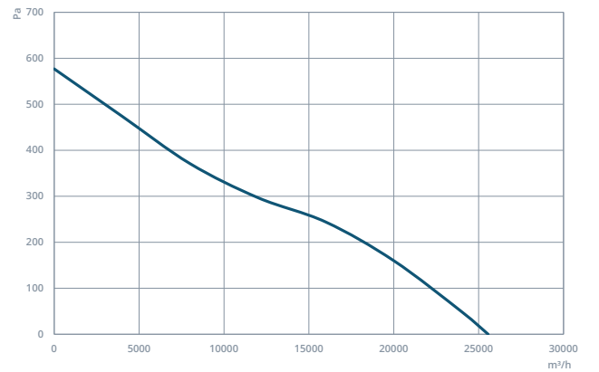
GAXI 800-5-30
