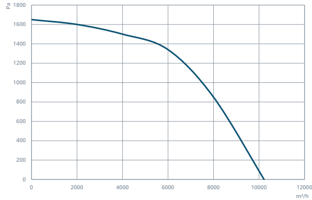
EC-CRAD 400
