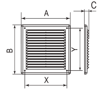
Genel boyutlar
