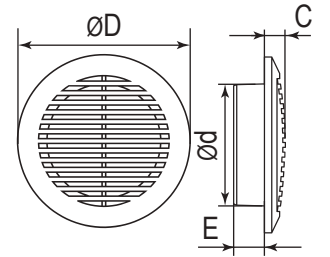
Genel boyutlar
