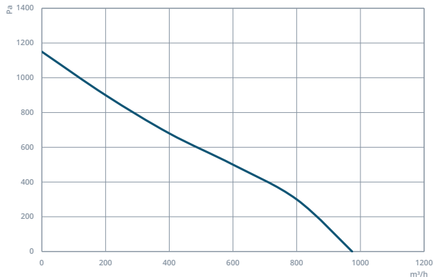
EC-CRAD 190
