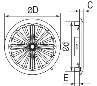
Genel boyutlar
