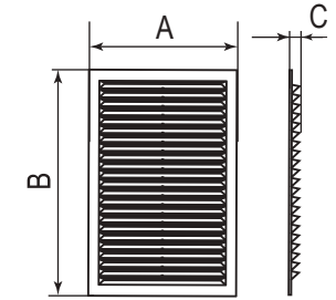
Genel boyutlar
