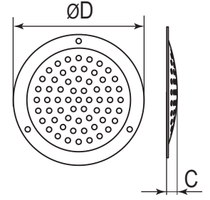
Genel boyutlar
