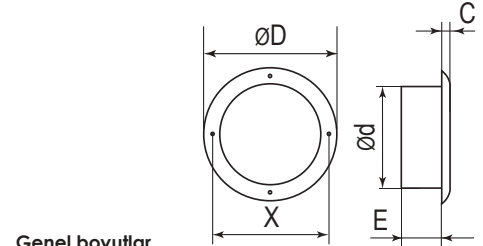
Genel boyutlar
